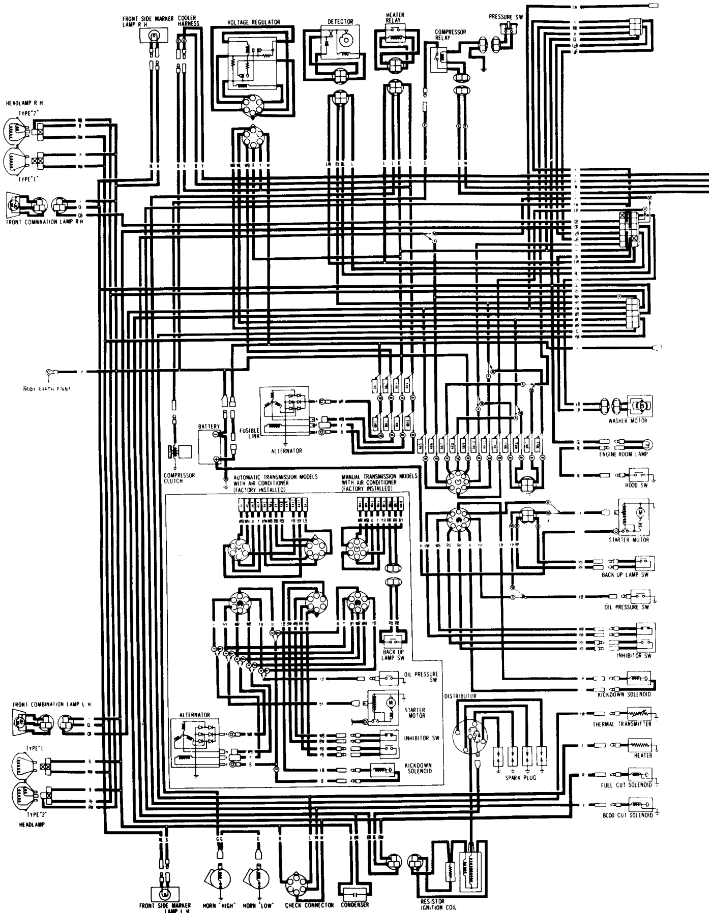
Fig. 10.38. Wiring diagram - 1975 USA
