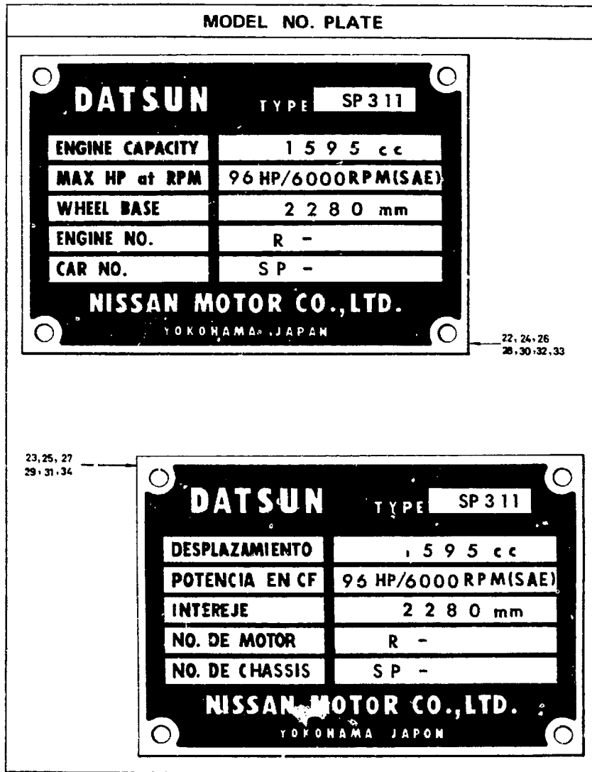
FIG. 62-3 B3 NISSAN MOTOR CO., LTD.
